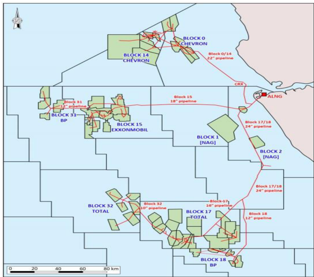
[NOTA: Os gasodutos entre os blocos não fornecedores são operados pela SOMG] Figura 3 - Rede de Gasodutos Upstream a Fábrica ALNG, no Soyo
