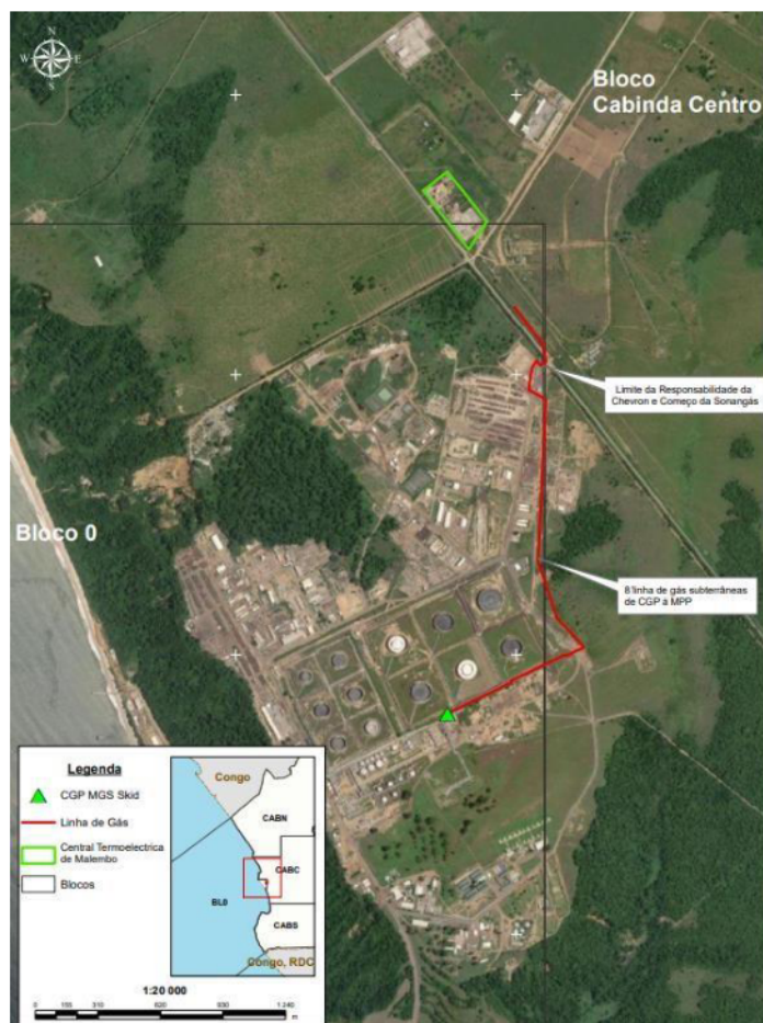
Figura 25 - Ponto de Entrada e ligação de gasodutos à Central Malembo em Cabinda, Fonte: ANPG.
