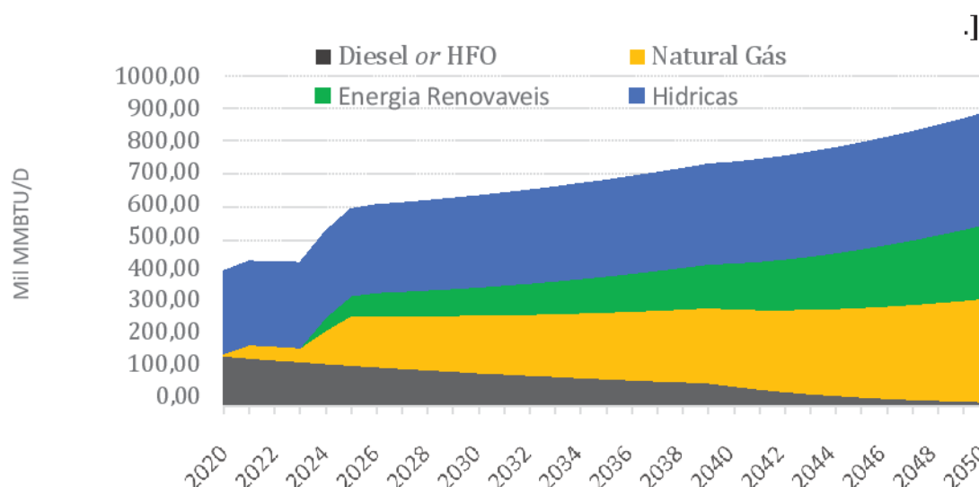
Gráfico 7 - Transição Energética: Ciclo da coabitação das várias fontes de energia (informação por analisar/validar MINEA, MIREMPET)
