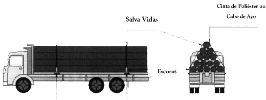
Sistema de sarilhos de amarração ou equivalente ajustável para amarração de cintas de poliéster ou cabos de aço.
